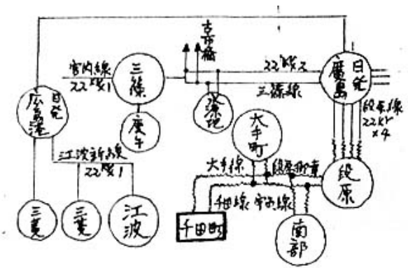
第9図 広島市附近送電系統図
