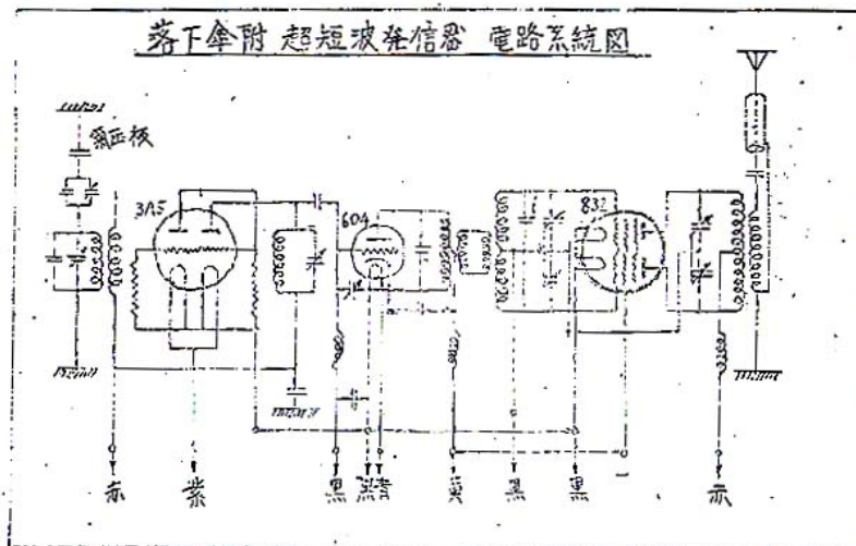
落下傘付超短波発信器 電路系統図
